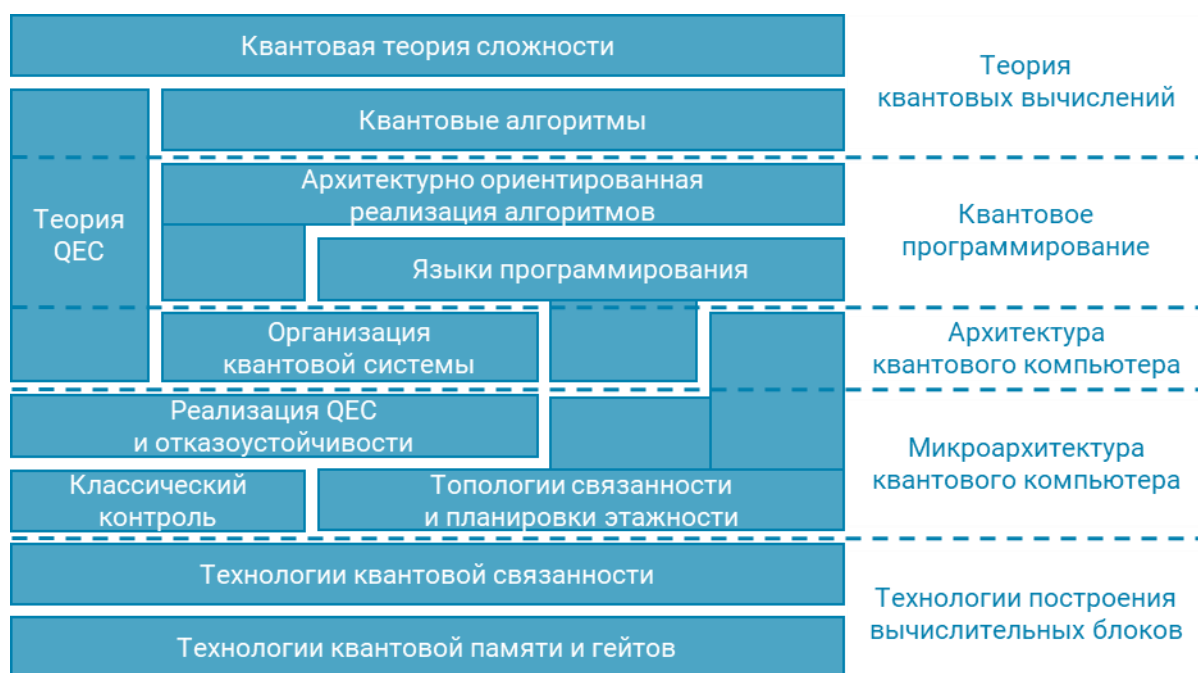
Рис.3. Основные направления развития квантовых технологий
