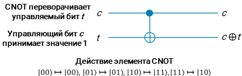
Рис. 2. Применение гейта (оператора) CNOT
